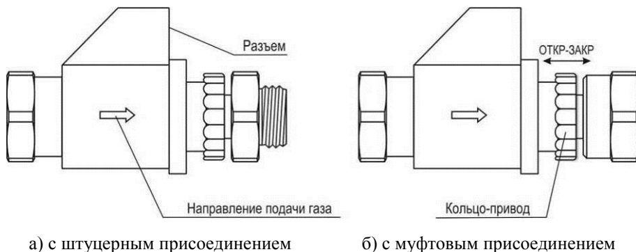
Рисунок 3 – Внешний вид клапана типа КЗЭУГ-Б
