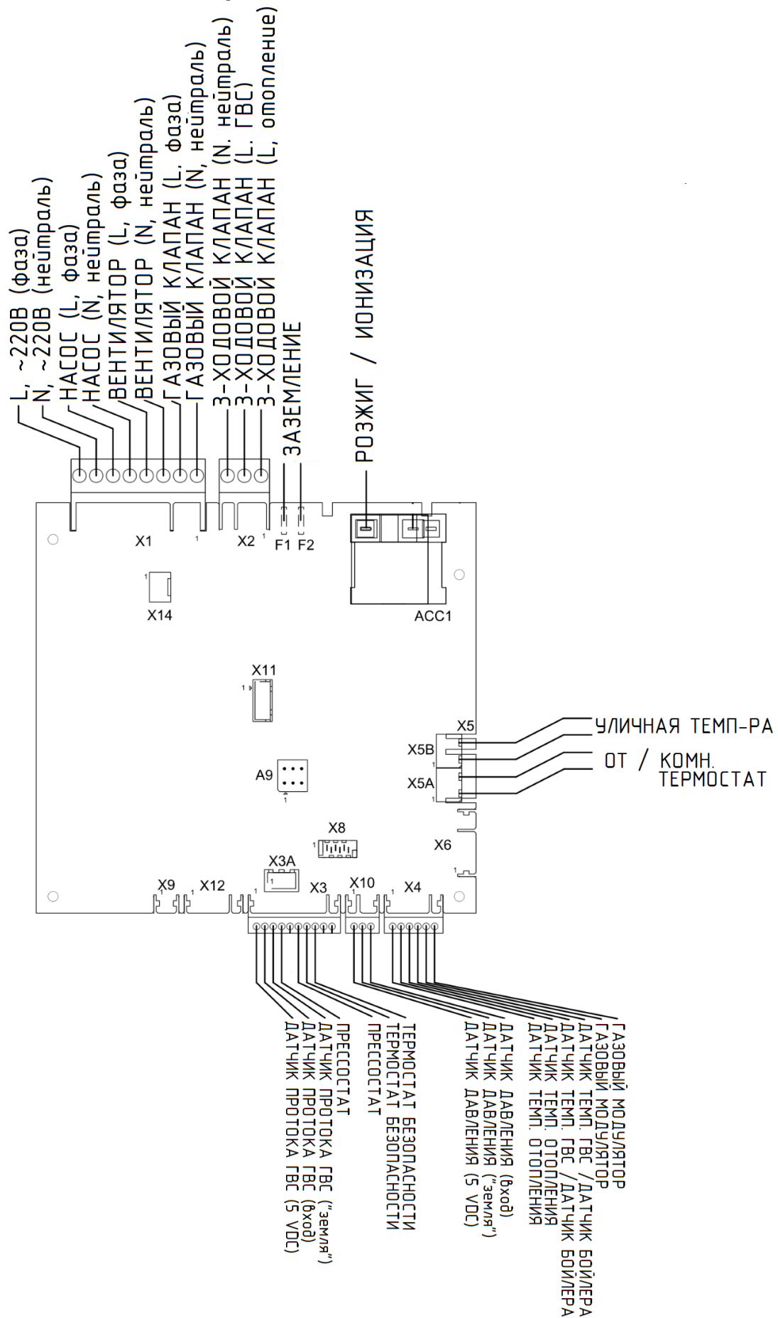
Рис. 13. Электрическая схема
