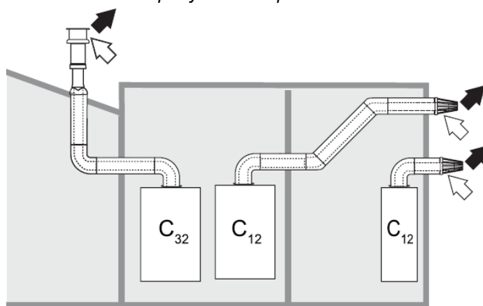
Рис. 7. Пример систем дымоудаления собранных с помощью коаксиальных труб. Белой стрелкой обозначен приток воздуха, чёрной стрелкой отвод продуктов сгорания.
