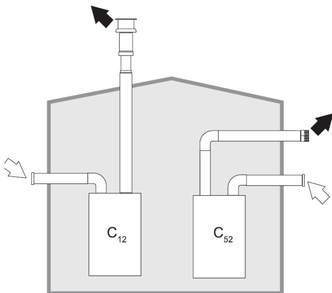
Рис. 4. Пример систем дымоудаления собранных с помощью отдельных труб. Белой стрелкой обозначен приток воздуха, чёрной стрелкой отвод продуктов сгорания
