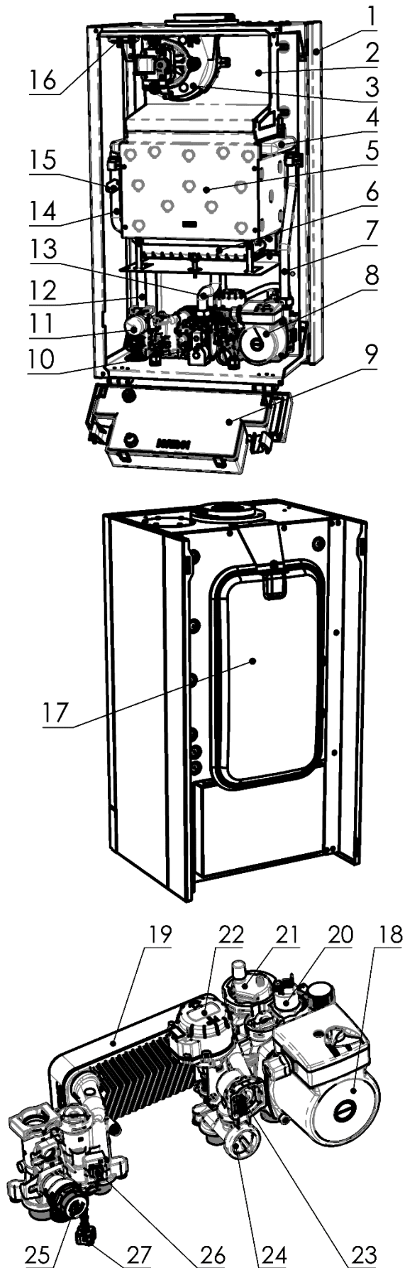
Рис. 10. Общая схема и основные элементы котла
