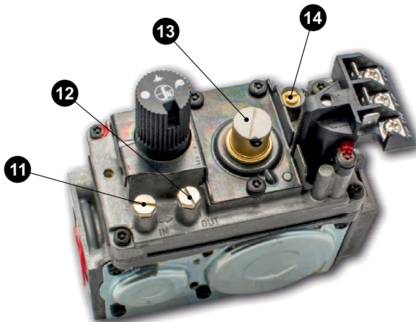
Рисунок 19. Элементы регулировки газового клапана SIT 820 NOVA mv
