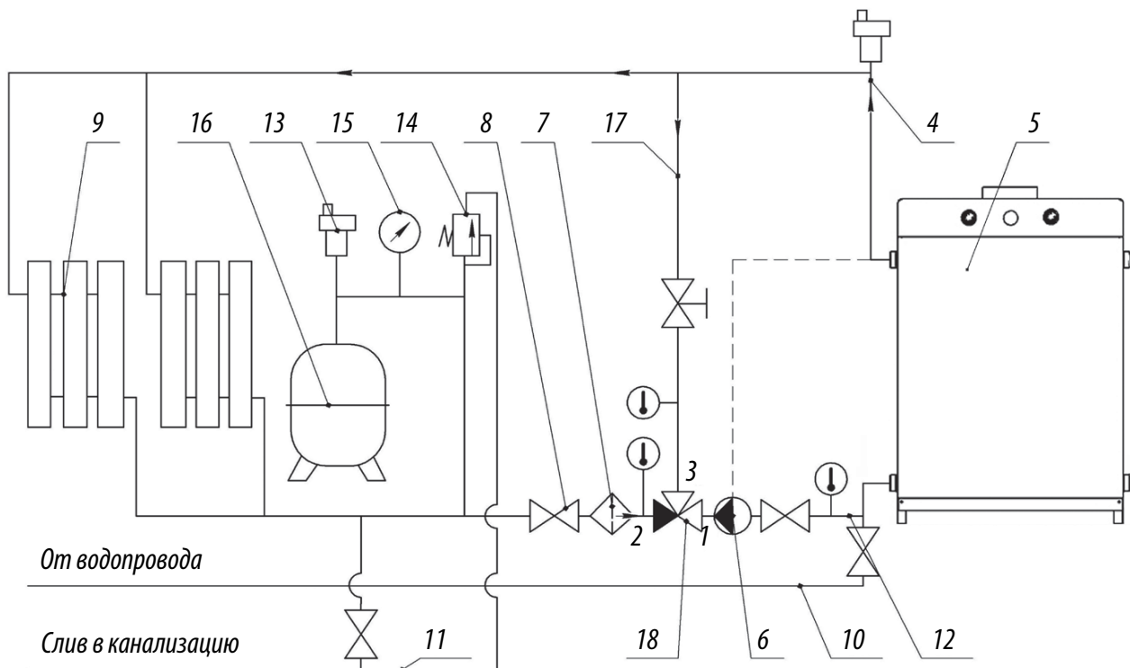
Рисунок 8 - Рекомендуемая гидравлическая закрытая схема системы отопления с байпасной линией рециркуляции, автоматическим трехходовым клапаном для прогрева теплоносителя в теплообменнике котла в целях исключения образования конденсата.
