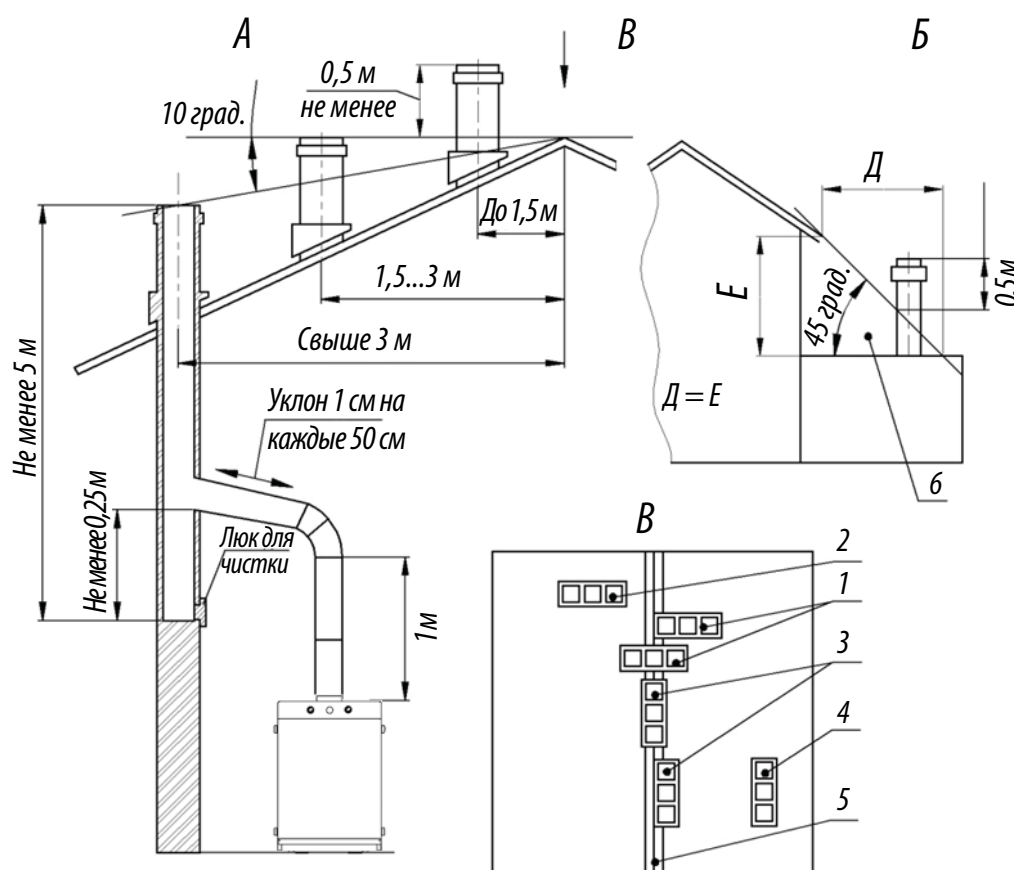
Рисунок 5. Схема расположения дымовой трубы
