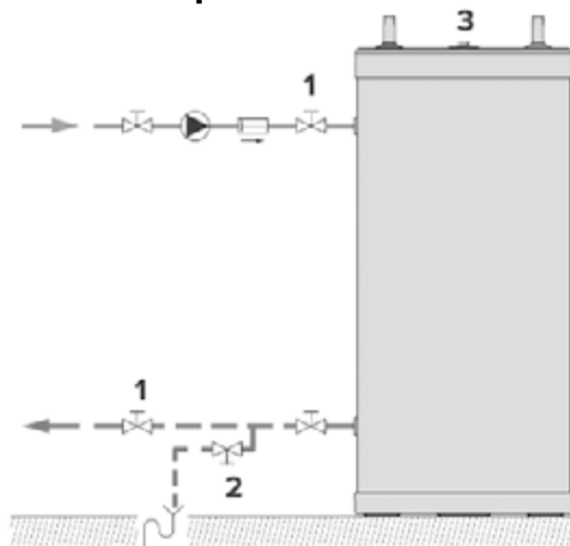
— — — Отвод теплоносителя к котлу — — — — — Подача теплоносителя в водонагреватель
