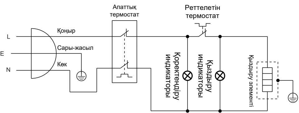
MQ1, MQ2 электр тізбегі
