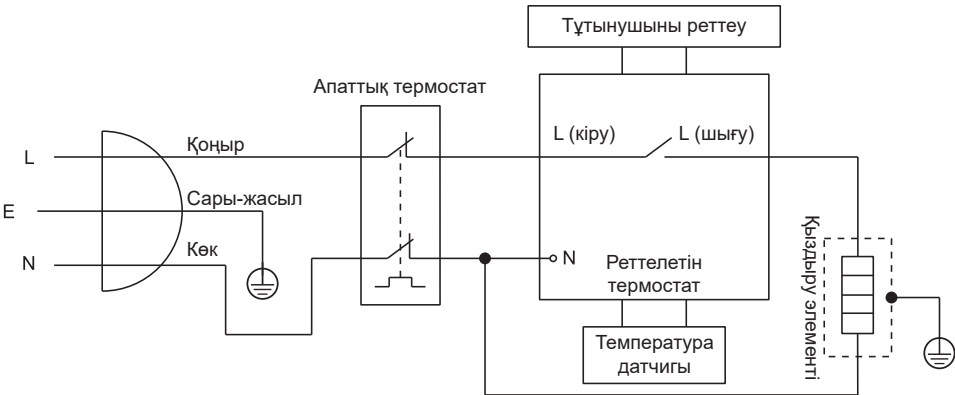
EQ1, EQ2 электр тізбегі
