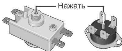
Рисунок 3. Схема расположения кнопки термовыключателя
