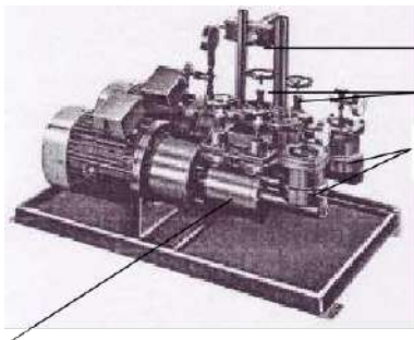
НАСОСНАЯ ГРУППА
