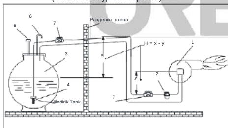
2-Х ТРУБНАЯ СЕТЬ
