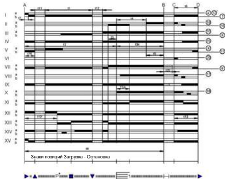
ВРЕМЕННАЯ ДИАГРАММА
