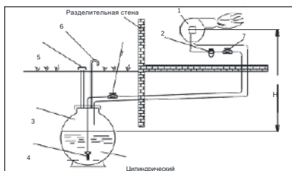
2-Х ТРУБНАЯ СЕТЬ
