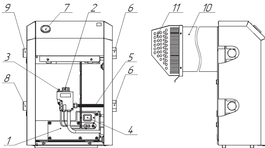
Рис. 1. Котёл «Патриот» с автоматикой 630 EUROSIT
