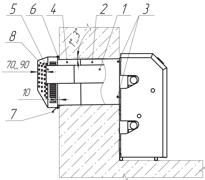
Рис. 2. Монтаж котла
